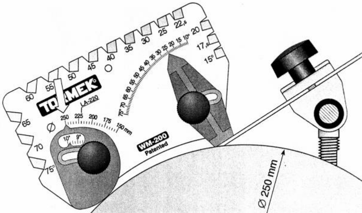
Nastavení želízka do hoblíku – úhel 25°, průměr kotouče 250mm, přípravek SE-77 (76)
