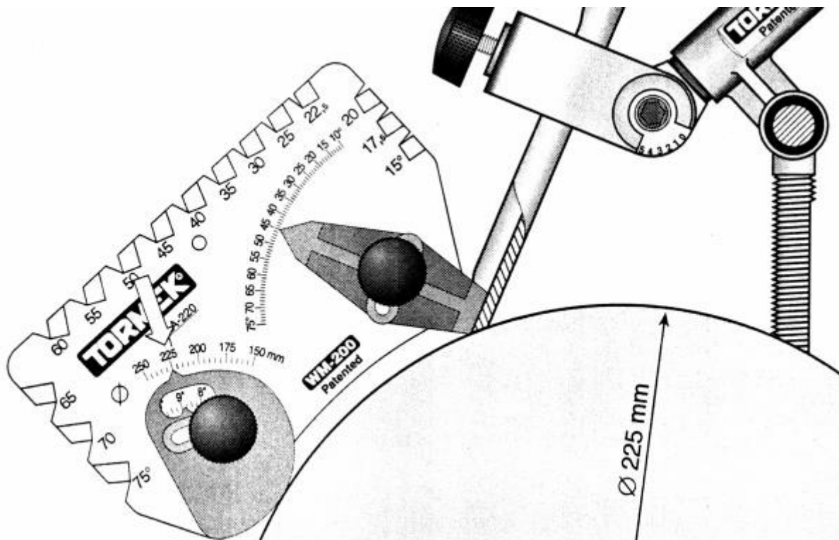
Nastavení úhlu kulatého dláta – úhel 45°, průměr kotouče 225 mm, přípravek SVD-186R (186)
